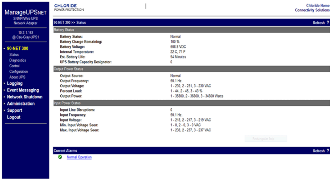
Hình 44: Hệ thống giám sát UPS của công ty
